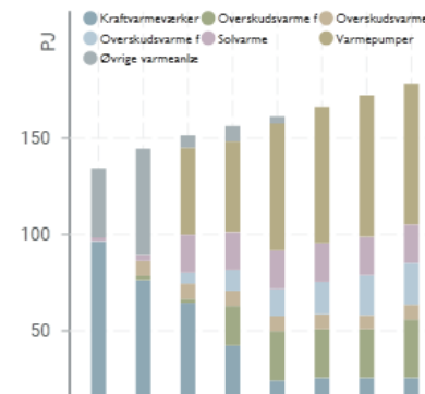
Fjernvarme-produktion
