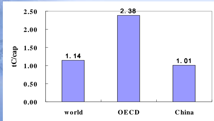
Per capita carbon emission
