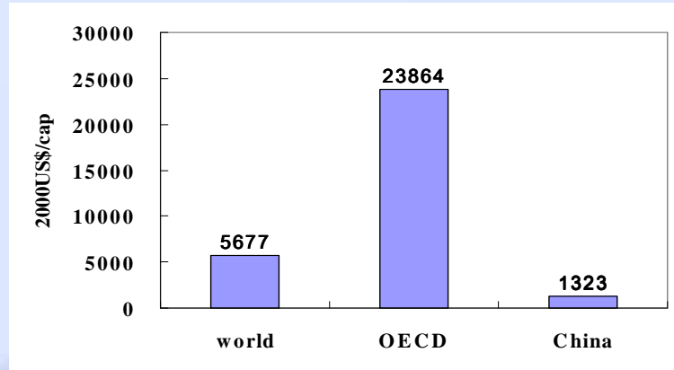
Per capita GDP
